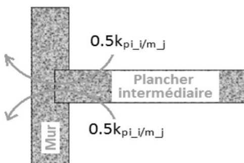
Ponts thermiques Plancher intermédiaire/Mur
